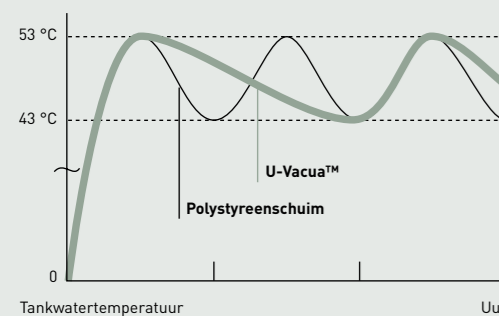
U-Vacua™: Vacuümislatiepaneel
