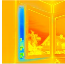
Geöffnetes Fenster (10 cm Spalt)
