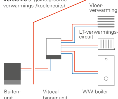
Versie 2C (2 geïntegreerde verwarmings-/koelcircuits)
